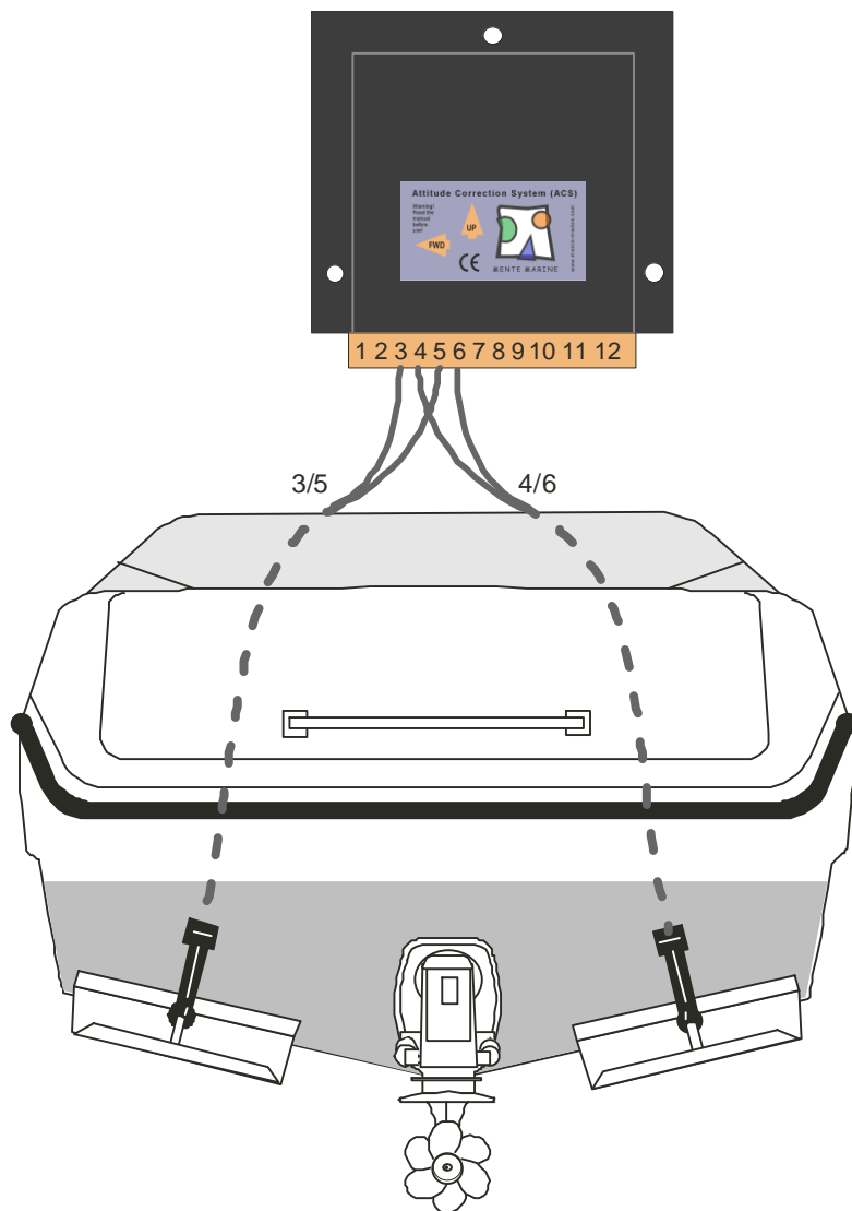
Inkoppling till elektromekaniska trimplan sett bakifrån
