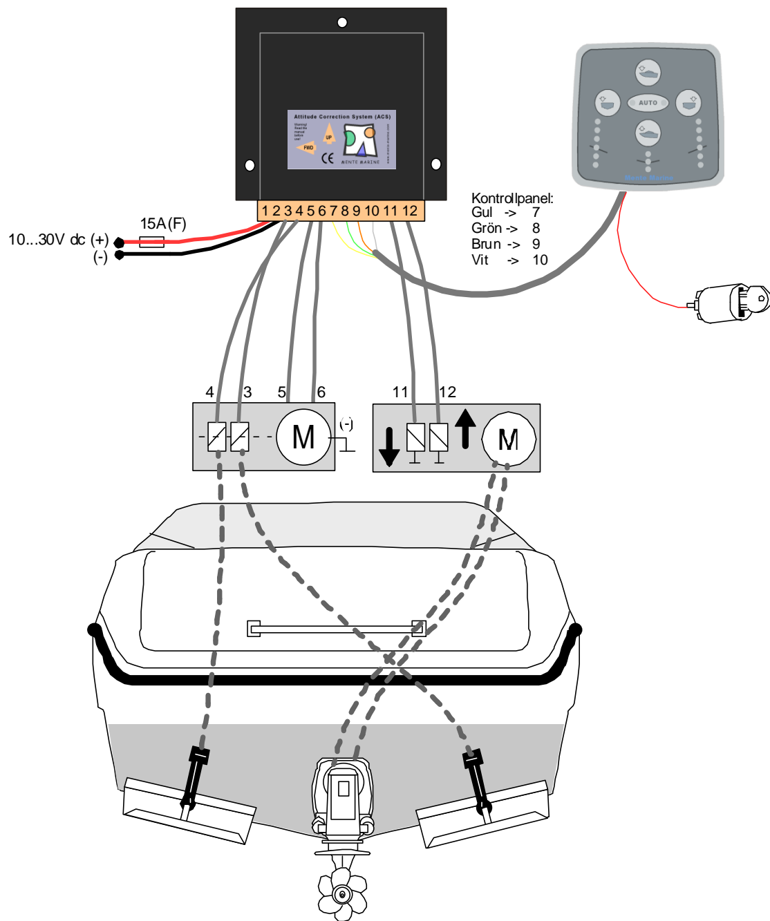
Inkoppling till hydrauliska trimplan och power trim sett bakifrån
