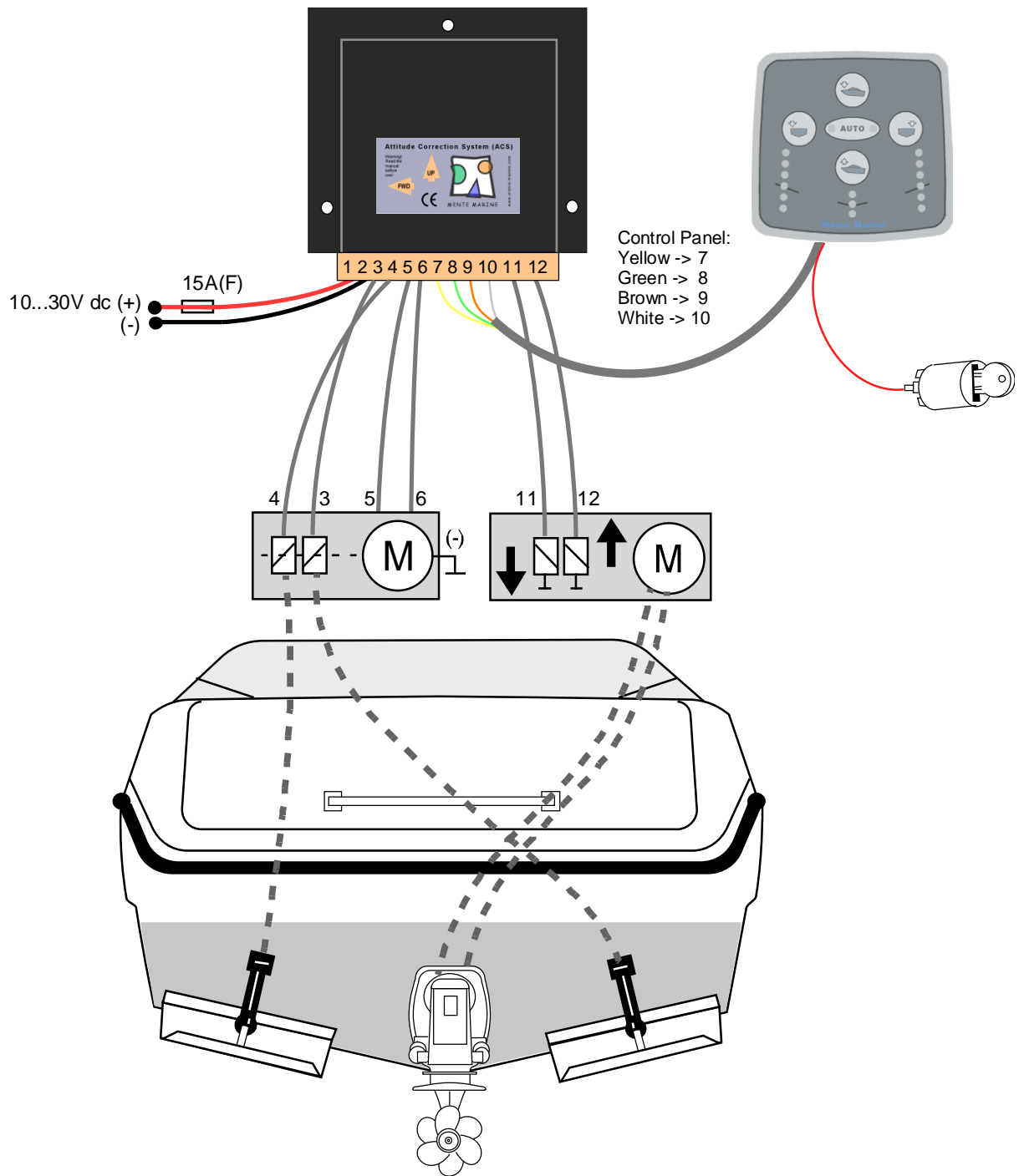
Bild 7. Anschluß der hydraulischen Trimmklappen und des Power Trim's. Blick in Fahrtrichtung
