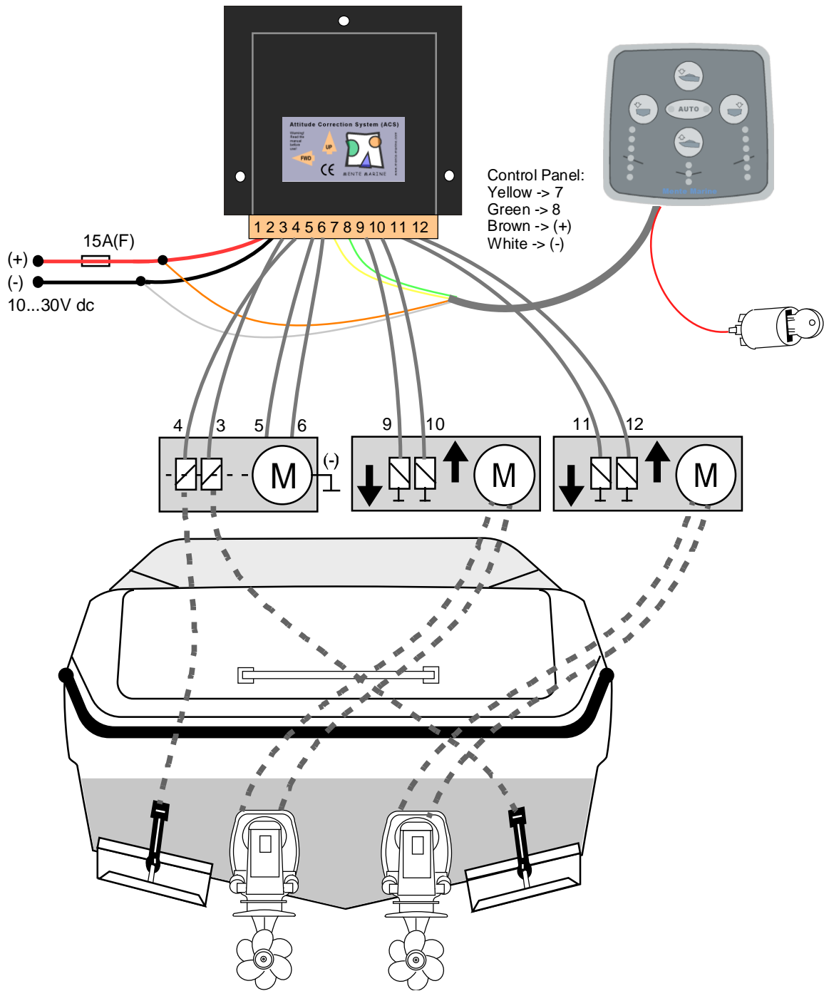
Bild 8. Anschluß der hydraulischen Trimmklappen und der Power Trim's bei zwei Motoren. Blick in Fahrtrichtung
