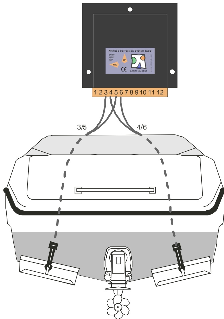
Bild 9. Anschluß der elektromechanischen Trimmklappen. Blick in Fahrtrichtung
