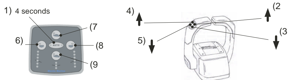
Bild 12. Tastenreihenfolge für die Kalibrierung
